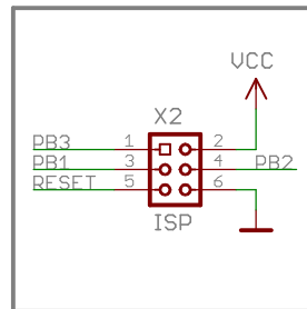
ISP_CONNECTOR
